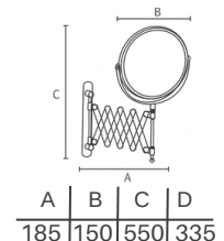
EP-L 6 Pantografico E6525
