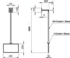
Porta Toalha IL 6830
