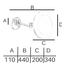
EF-L 8 c/ Luz E6510
