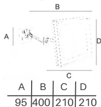
EF-L 9 c/ Luz E6505
