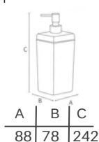
Porta Sabão Líquido Jateado
