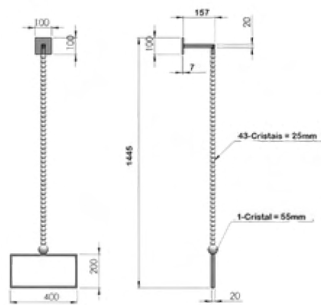
Porta Toalha IL 6820
