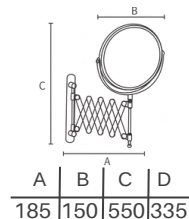
EP-F 6 Pantografico E6575
